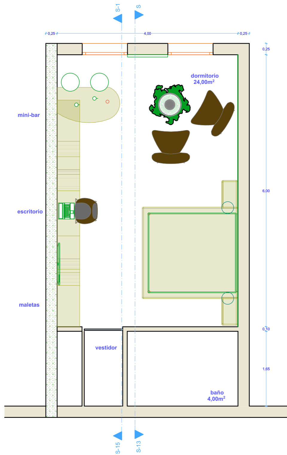
0. PLANTA 1:50
