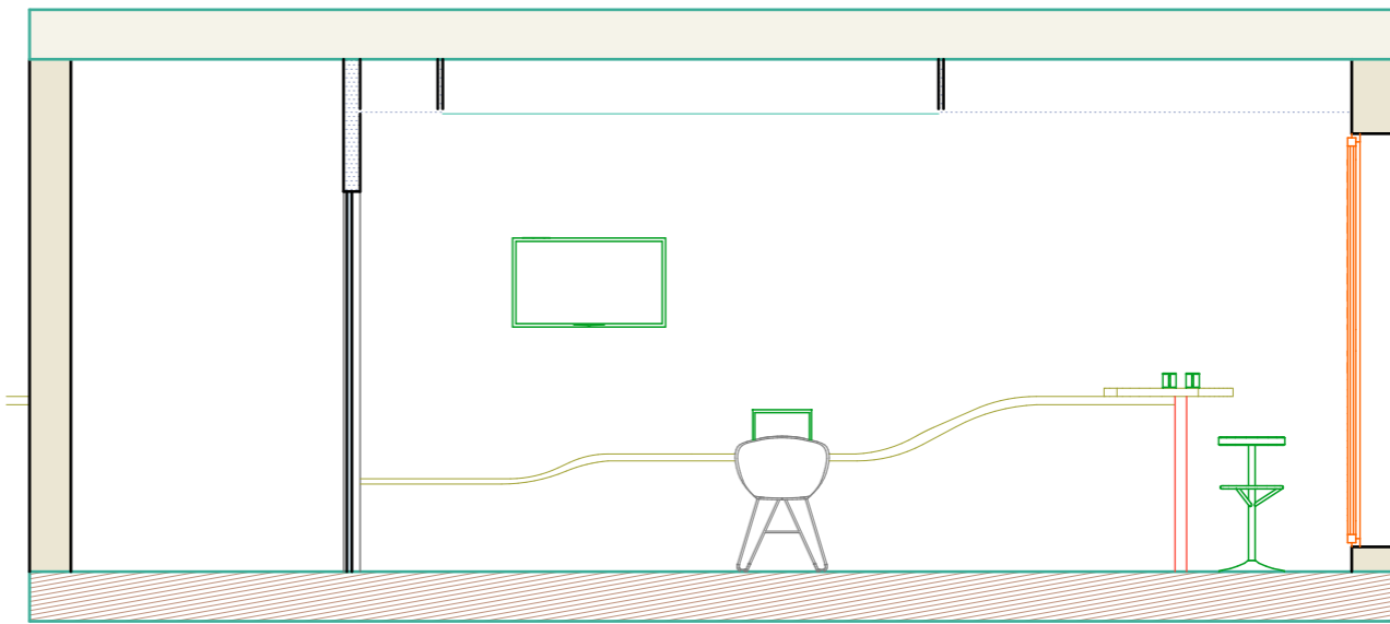
S-13 Sección Construcción (1) 1:50
