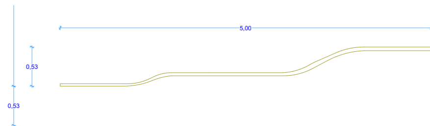
detalle tablero 1:50
